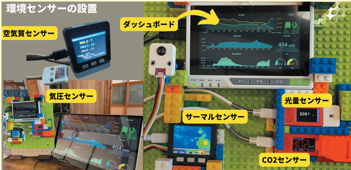
写真/佐々木博さん作、環境センサー
